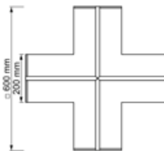
Kreuzungs-Element 1-läufig
