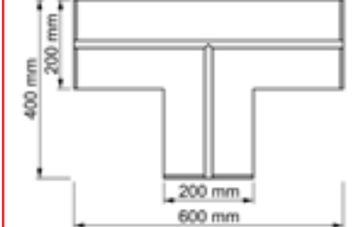
T-Element 1-läufig
